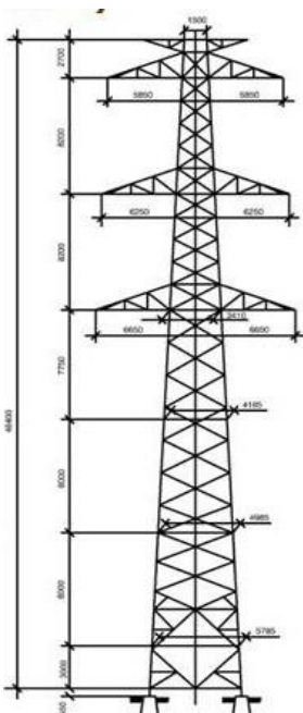
16. ábra: „Fenyő” oszlopkép. (Forrás: MAVIR)
