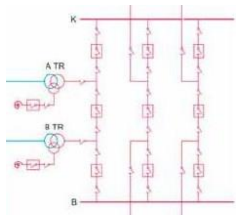
15. ábra: Másfél megszakítós diszpozíció. (Forrás: MAVIR)
